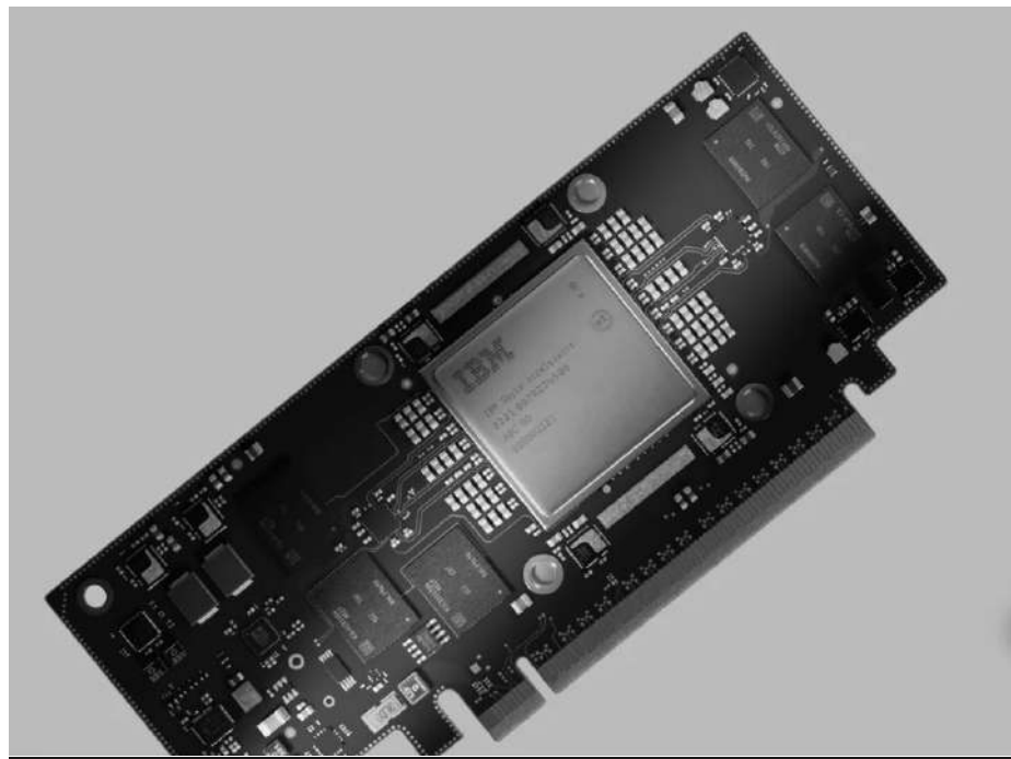
L'accélérateur IA Spyre embarque 32 cœurs d'accélérateur individuels et contient 25,6 milliards de transistors. Les cartes peuvent être regroupées - par exemple, un groupe de 8 cartes ajoute 256 cœurs d'accélération supplémentaires à un seul système IBM Z.
