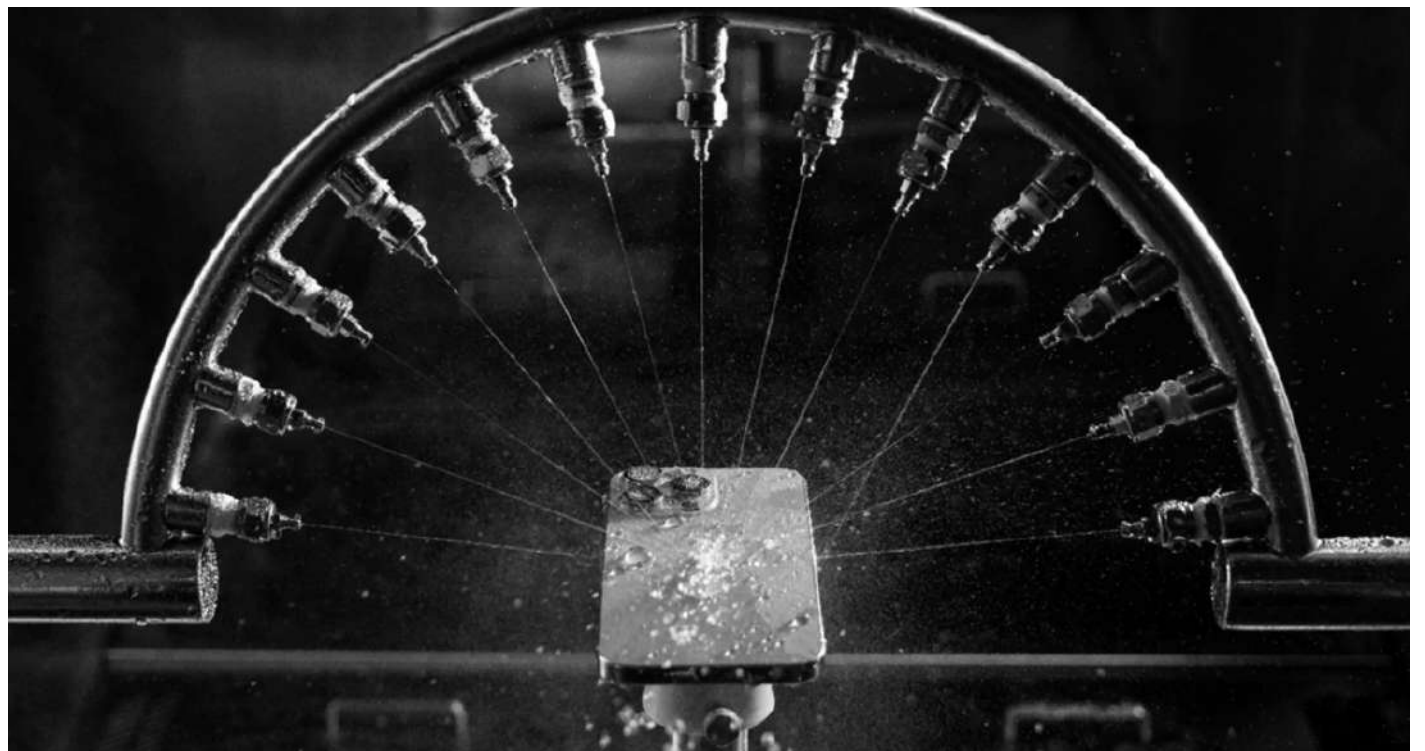
Un iPhone testé pour sa résistance aux infiltrations d'eau
