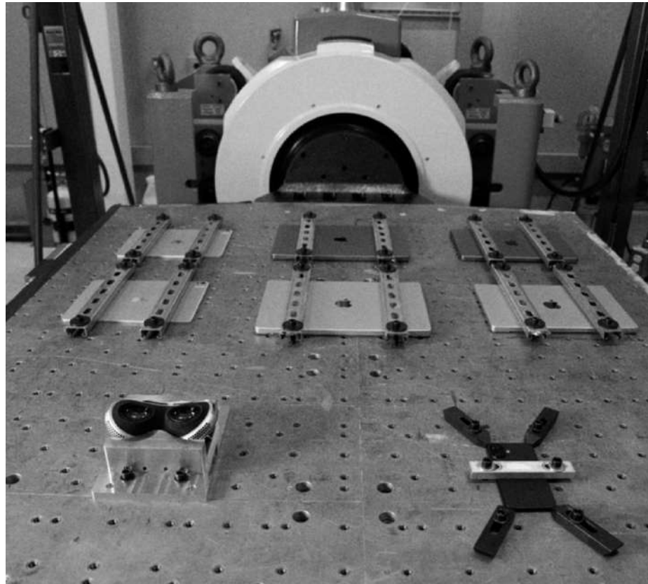
Différents appareils Apple testés pour leur résistance aux secousses sur une table vibrant
